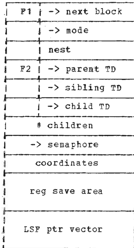
A Task Display
